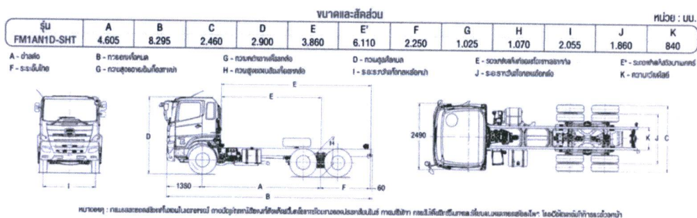
รูปที่ ๑ ตัวอย่างมิติรถบรรทุก ๑๐ ล้อ ยี่ห้อ HINO Vector ๕๐๐
