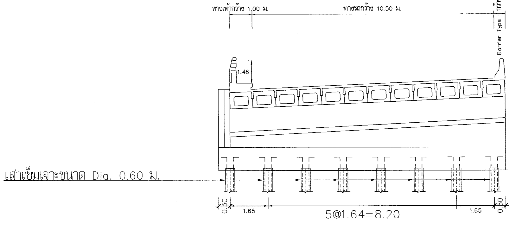
รูปตัดสะพาน A-A ขนาด 1:125
