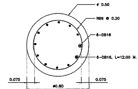
SECTION 2 - 2 SCALE 1 : 10
