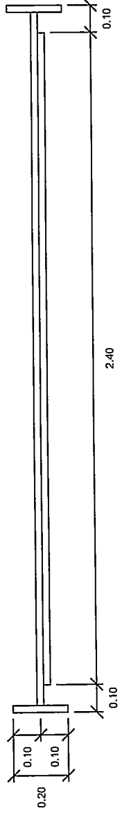
แปลน 1 : 50
