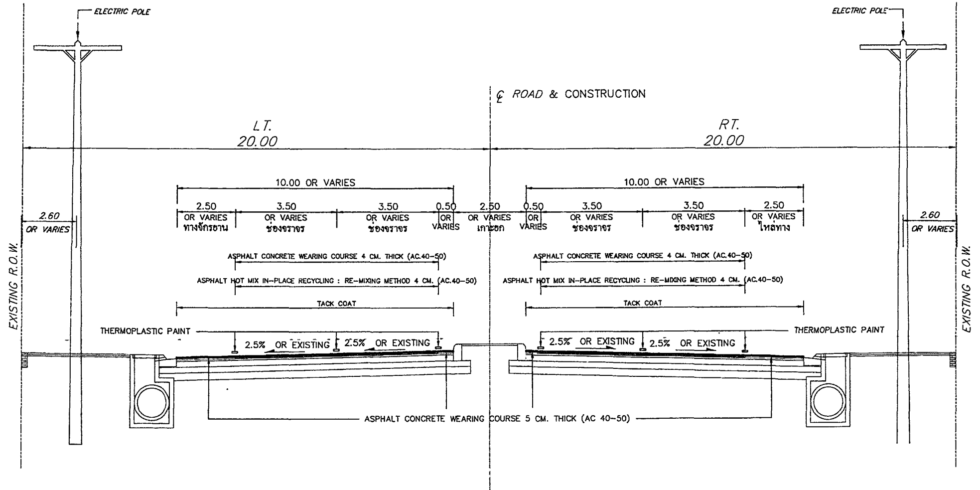
รูปตัดหลังดำเนินการ ระหว่าง กม.๕๓+๒๓๗ - กม.๕๓+๓๐๐
