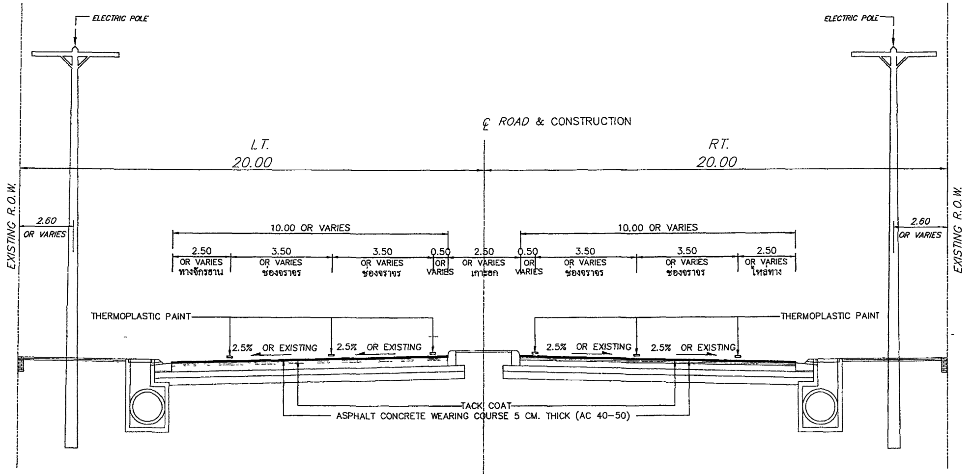
รูปตัดหลังดำเนินการ ระหว่าง กม.53+700 - กม.54+115
