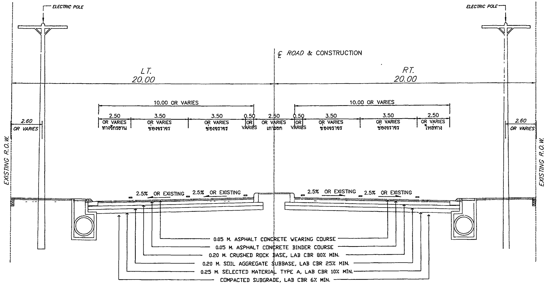
รูปตัดก่อนดำเนินการ
