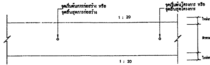
รายละเอียดแปลนบริเวณจุดเริ่มต้นหรือจุดสิ้นสุดการก่อสร้าง
