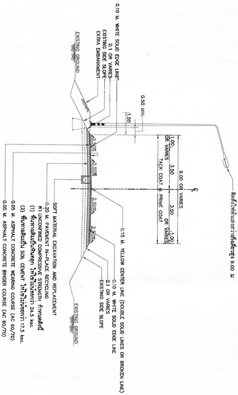
TYPICAL CROSS SECTION (หลังปรับปรุง)
