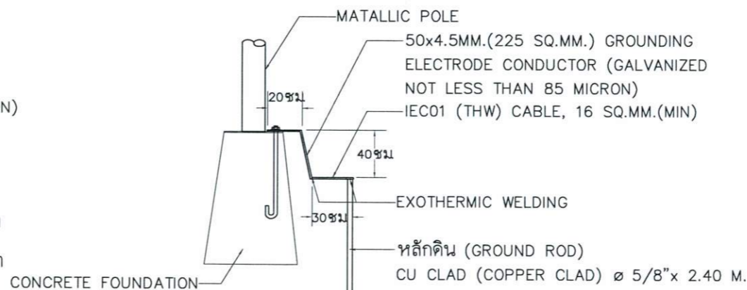
รูปที่ 1 แบบขยายการต่อ GROUND ROD
