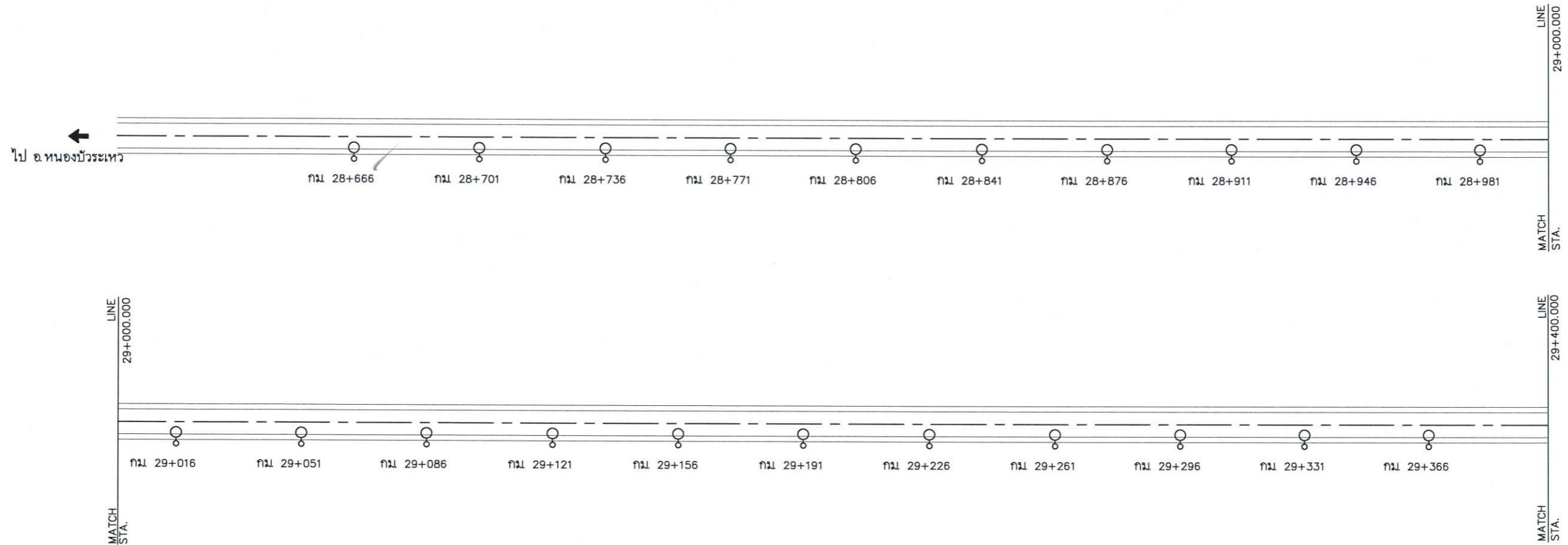
แบบแนะนำตำแหน่งติดตั้งไฟฟ้าแสงสว่าง NOT TO SCALE
