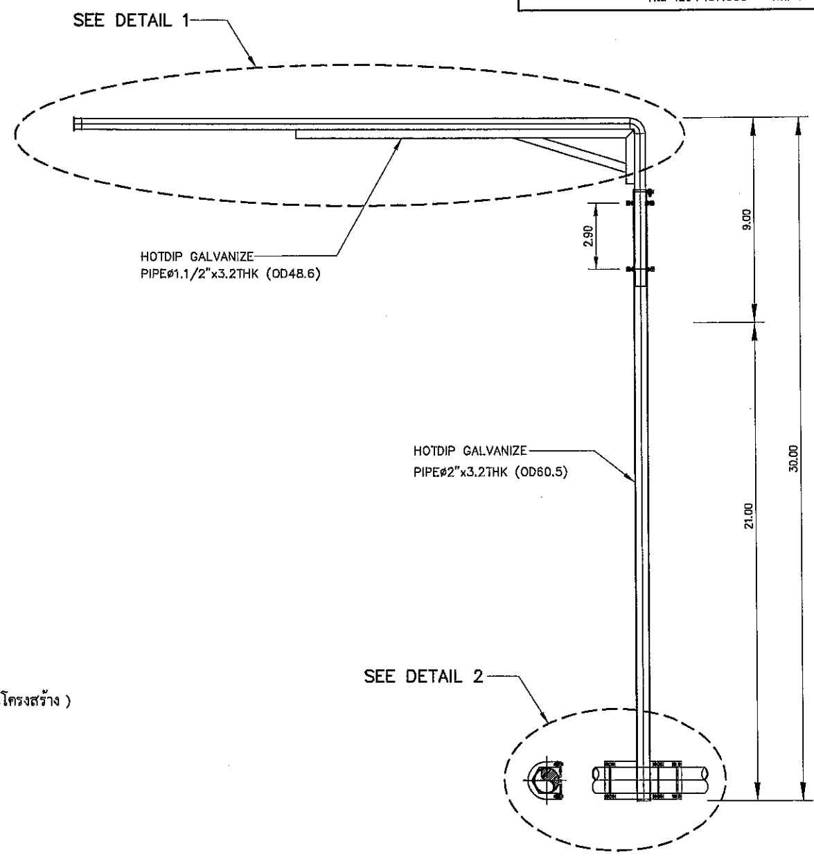
เสากล้องนับปริมาณจราจร NOT TO SCALE
