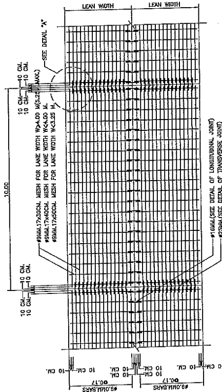
รูปที่ 1 การเสริมเหล็กกันรั่วงานคอนกรีตหนา 25 ซม.
