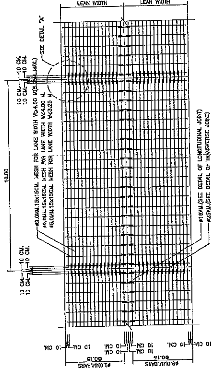
รูปที่ 2 การเสริมเหล็กตัวดัดตะแกรง wire mesh กันรั่วงานคอนกรีตหนา 25 ซม.
