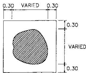
PLAN ขอบเขตการขุดตัด
