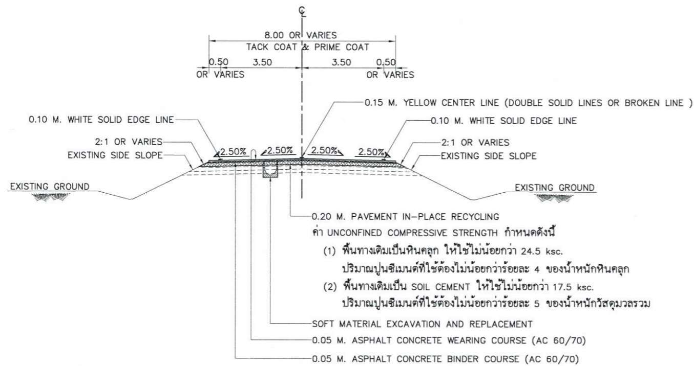
TYPICAL CROSS SECTION (หลังปรับปรุง) NOT TO SCALE กม. 9+526.000 - กม. 10+565.000
