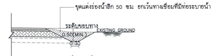
ทางเชื่อมถมเต็ม
