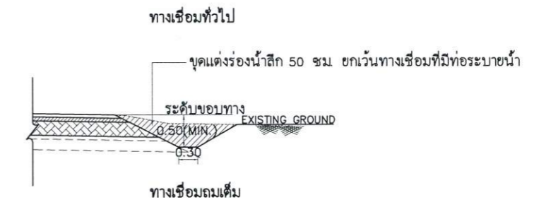
แบบขยายการปรับปรุงระบบระบายน้ำข้างทาง NOT TO SCALE
