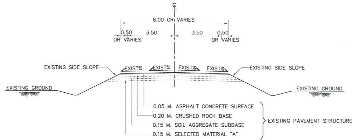
TYPICAL CROSS SECTION (ก่อนปรับปรุง) NOT TO SCALE กม. 9+526.000 - กม. 10+565.000
