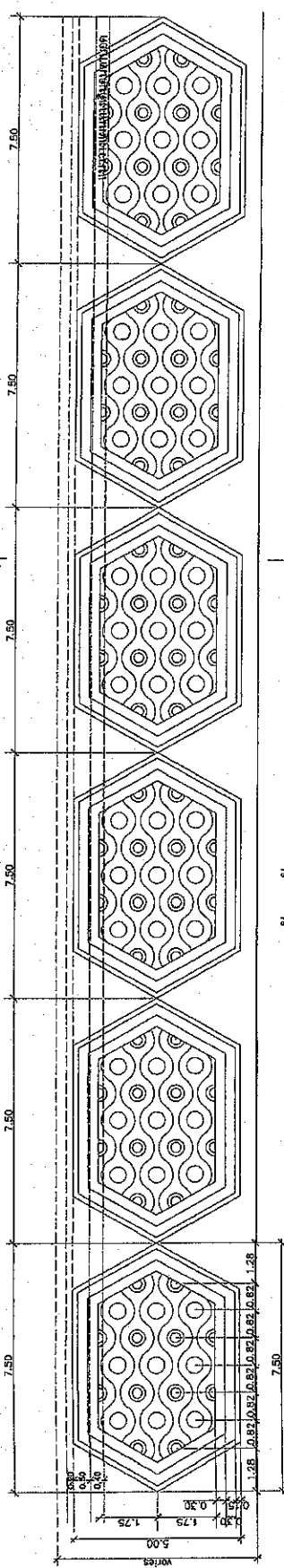
แปลน-ลายพื้นกว้าง > 5 เมตร
