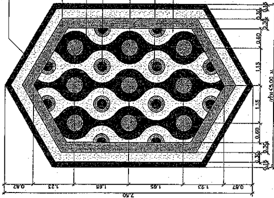
แบบขยาย รูปแบบที่ 4 ขนาด 1:25 (ลายพื้นกว้าง > 5.00 ม.)
