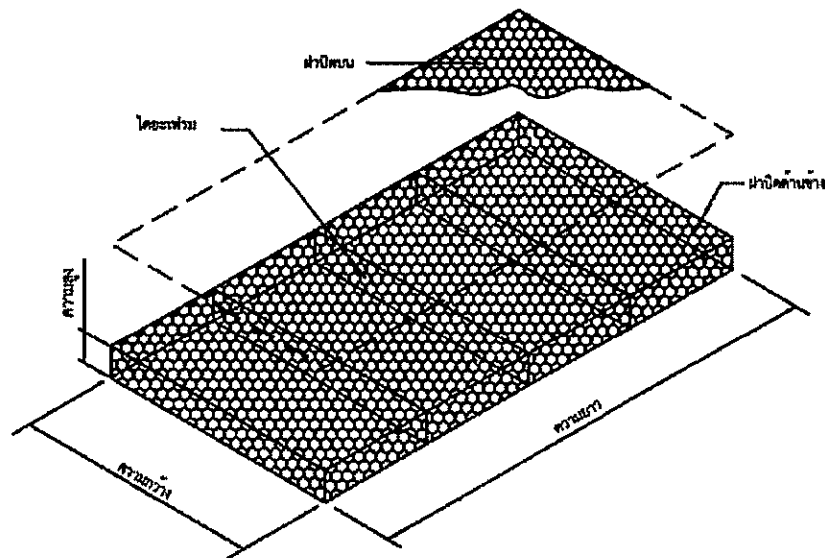
รูปที่ 1. แสดงขนาดมิติของกล่องลวดตาข่ายแมทเทรส (MATTRESS)
