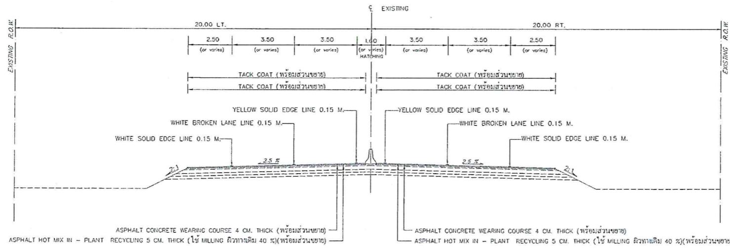
TYPICAL CROSS SECTION ระหว่าง กม.959+233 - กม.960+300 (LT.,RT.) (หลังปรับปรุง) SCALE 1:200
