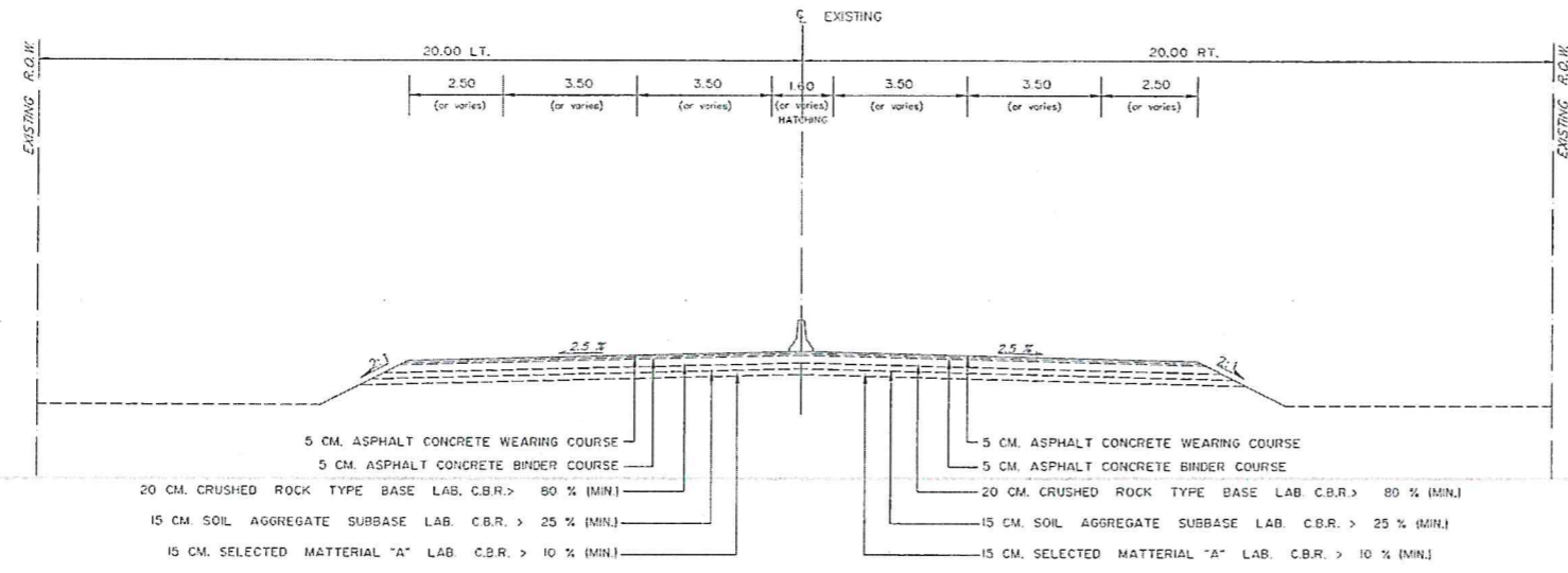
TYPICAL CROSS SECTION ระหว่าง กม.959+233 - กม.960+300 (LT.,RT.) (ก่อนปรับปรุง) SCALE 1:200
