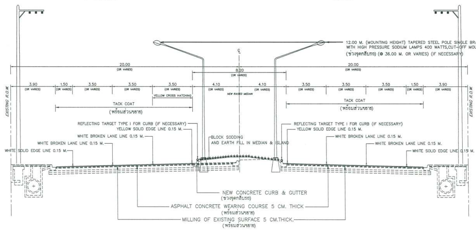
TYPICAL CROSS SECTION ทล.402 ระหว่าง กม.36+194 - กม.36+714 (ก่อนปรับปรุง) SCALE 1:200
