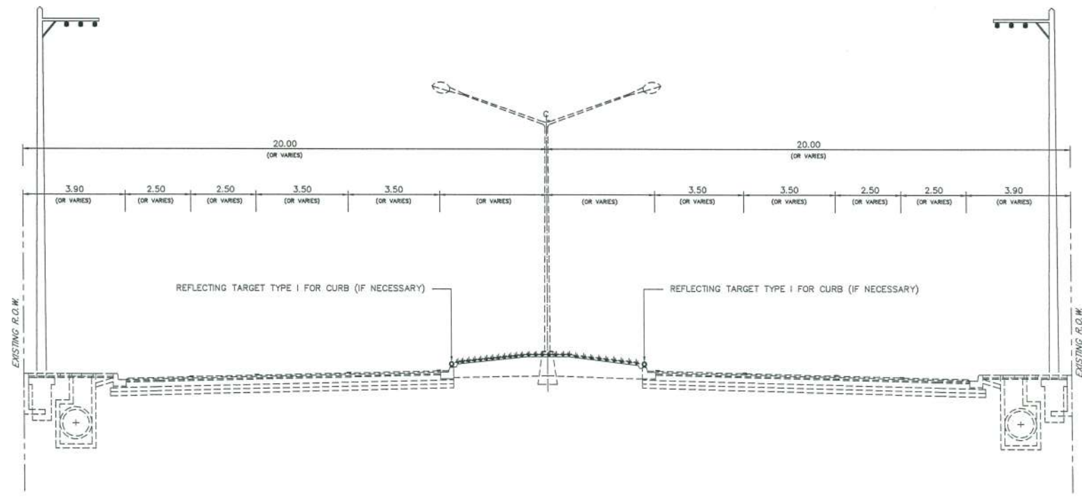
TYPICAL CROSS SECTION ทล.402 ระหว่าง กม.36+790 - กม.36+925 (ก่อนปรับปรุง) SCALE 1: 200
