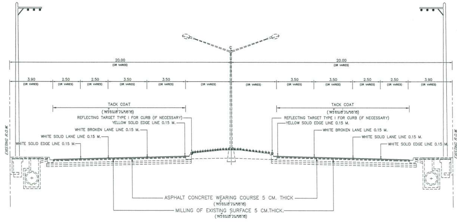
TYPICAL CROSS SECTION ทล.402 ระหว่าง กม.36+714 - กม.36+790 (ก่อนปรับปรุง) SCALE 1: 200
