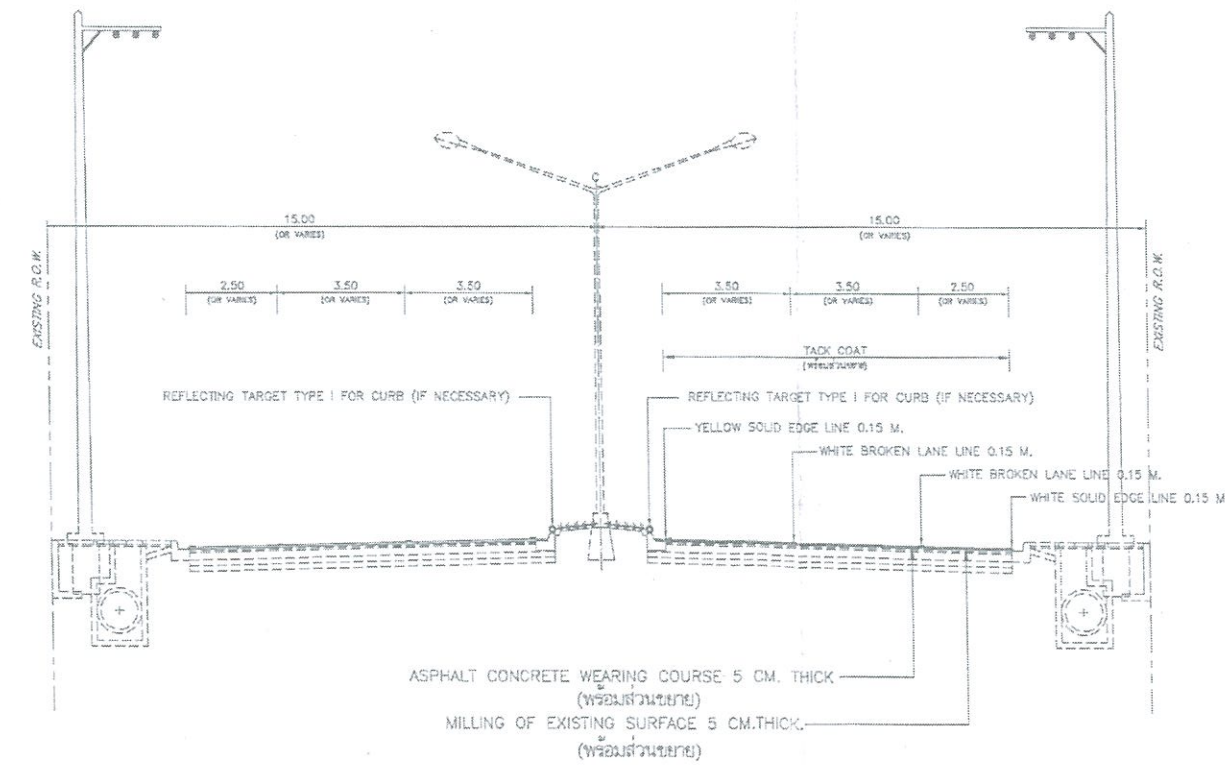
TYPICAL CROSS SECTION ทล. 402 ระหว่าง กม.31+438 - กม.31+550 RT. (ก่อนปรับปรุง) SCALE 1:200
