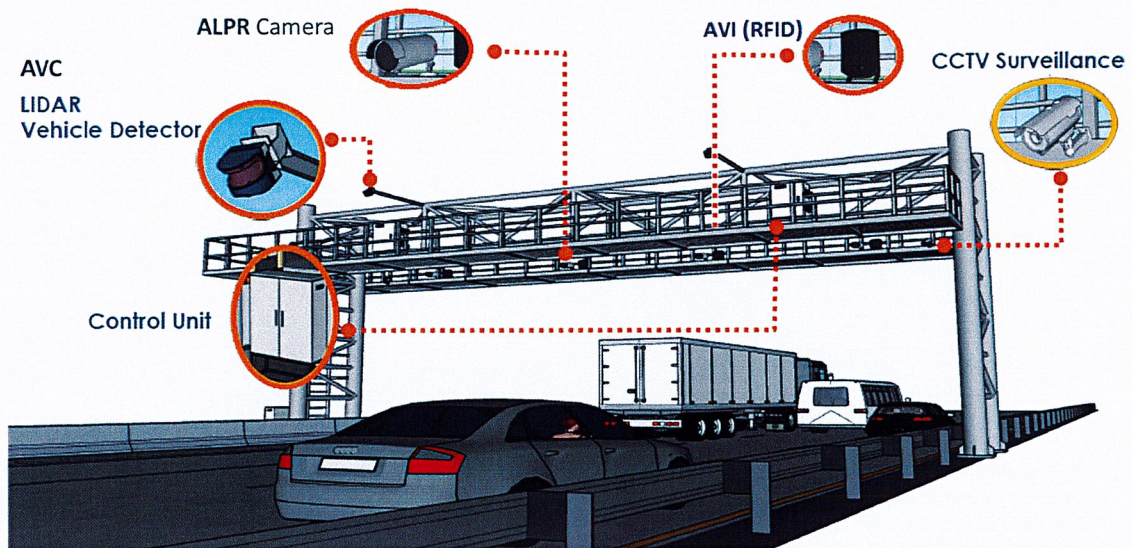
รูปที่ ๑.๒-๔ ตัวอย่างรูปแบบการติดตั้งอุปกรณ์และโปรแกรมระบบในระดับช่องทาง (Lane) ของระบบ M-Flow ในรูปแบบ MLFF
