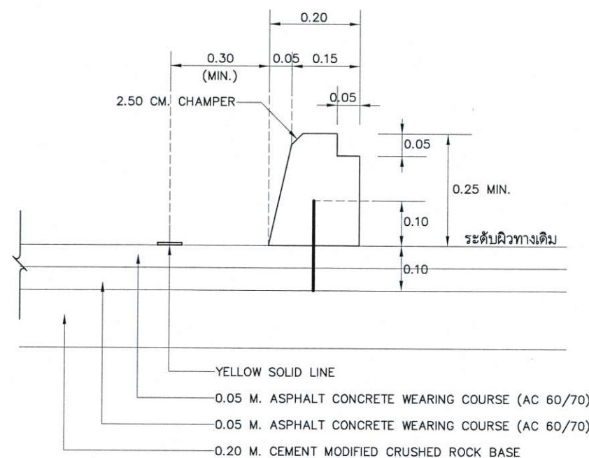
แบบขยาย ① CONCRETE CURB 0.25 M. THICK
