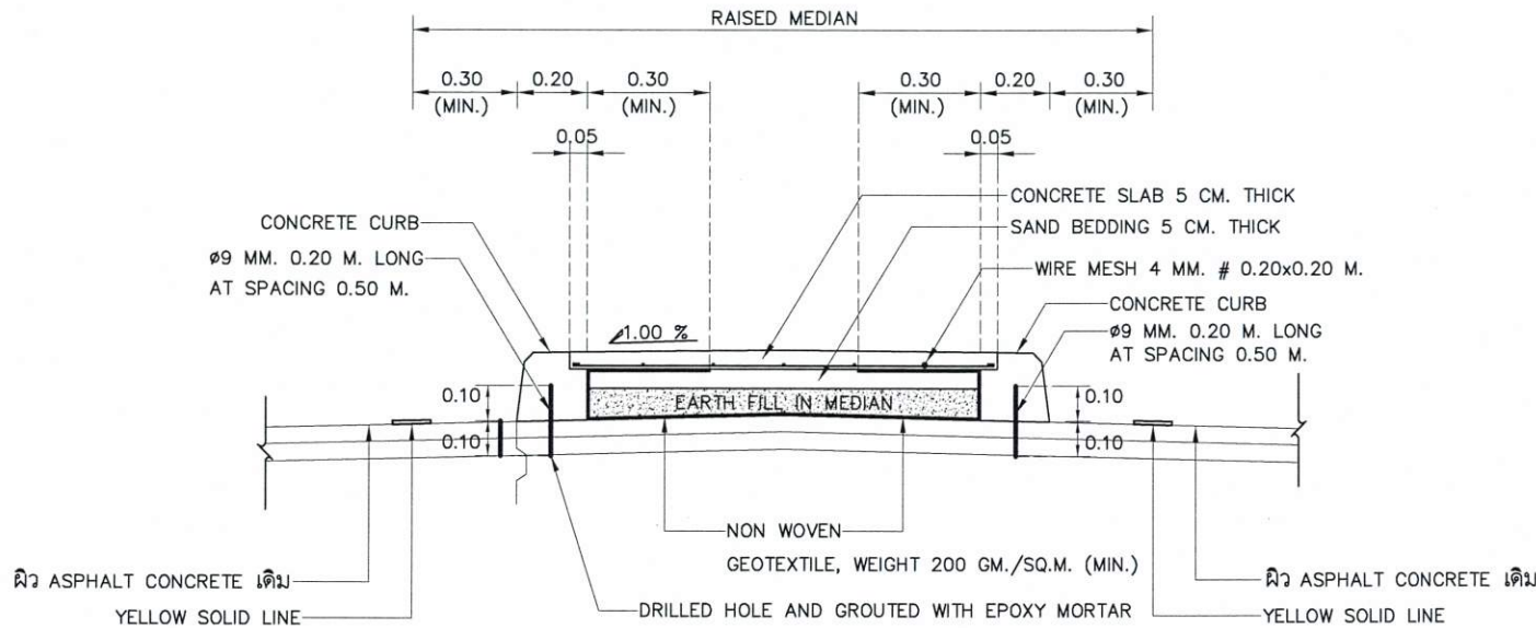
แบบขยาย ② RAISED MEDIAN ON EXISTING PAINTED MEDIAN
