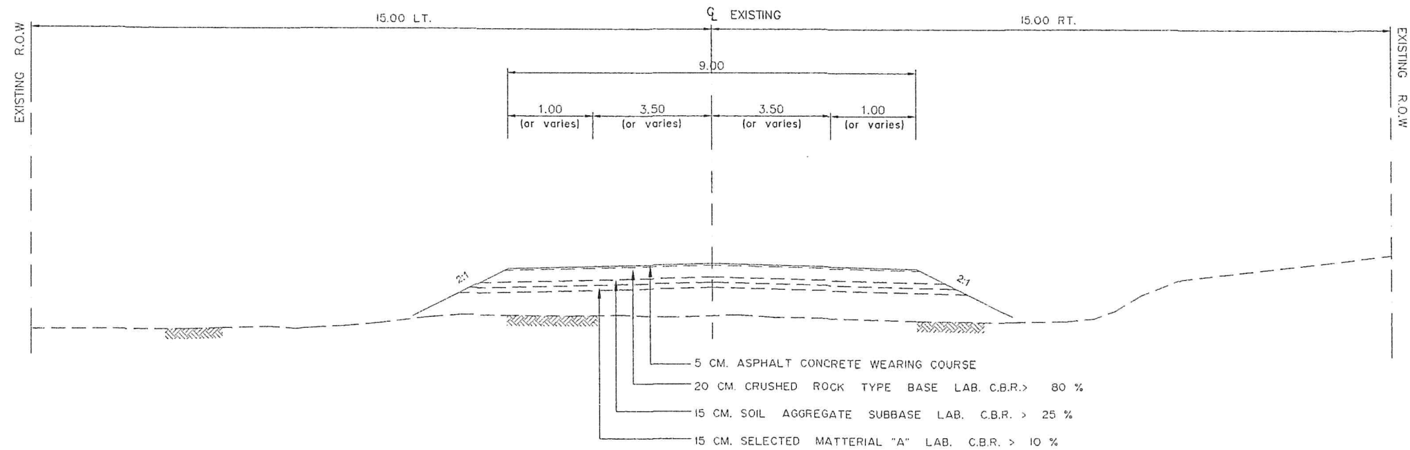
TYPICAL CROSS SECTION ระหว่าง กม.8+000 - กม.10+822 (LT.)(ก่อนปรับปรุง) SCALE 1:200
