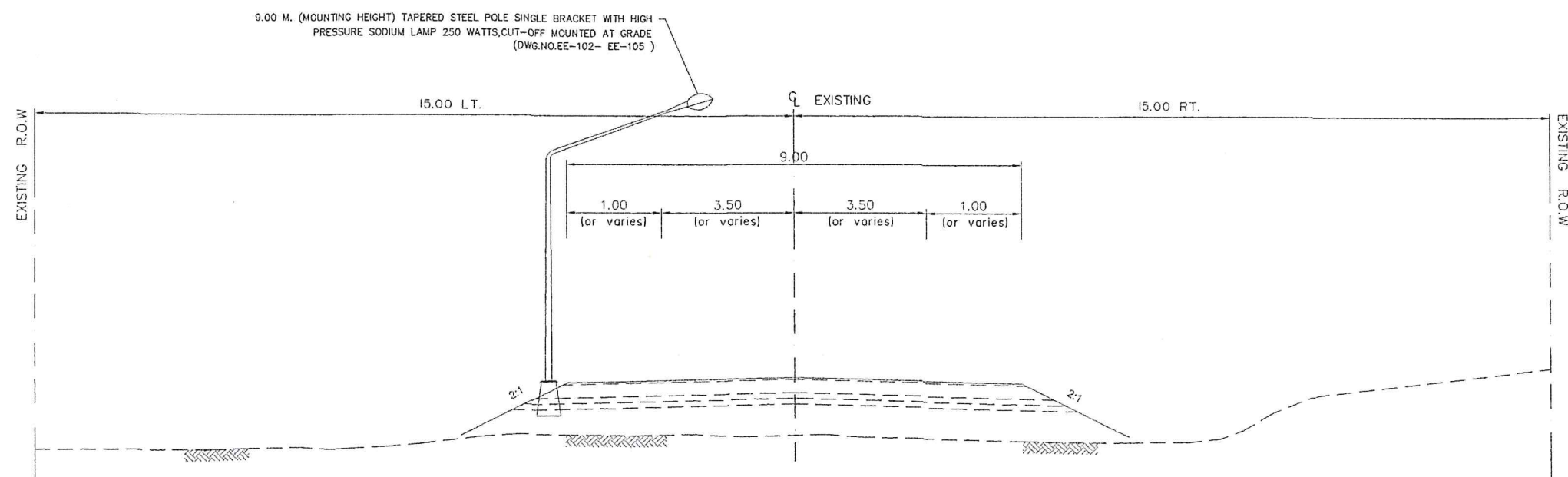
TYPICAL CROSS SECTION ระหว่าง กม.8+000 - กม.10+822 (LT.)(ก่อนปรับปรุง) SCALE 1:200
